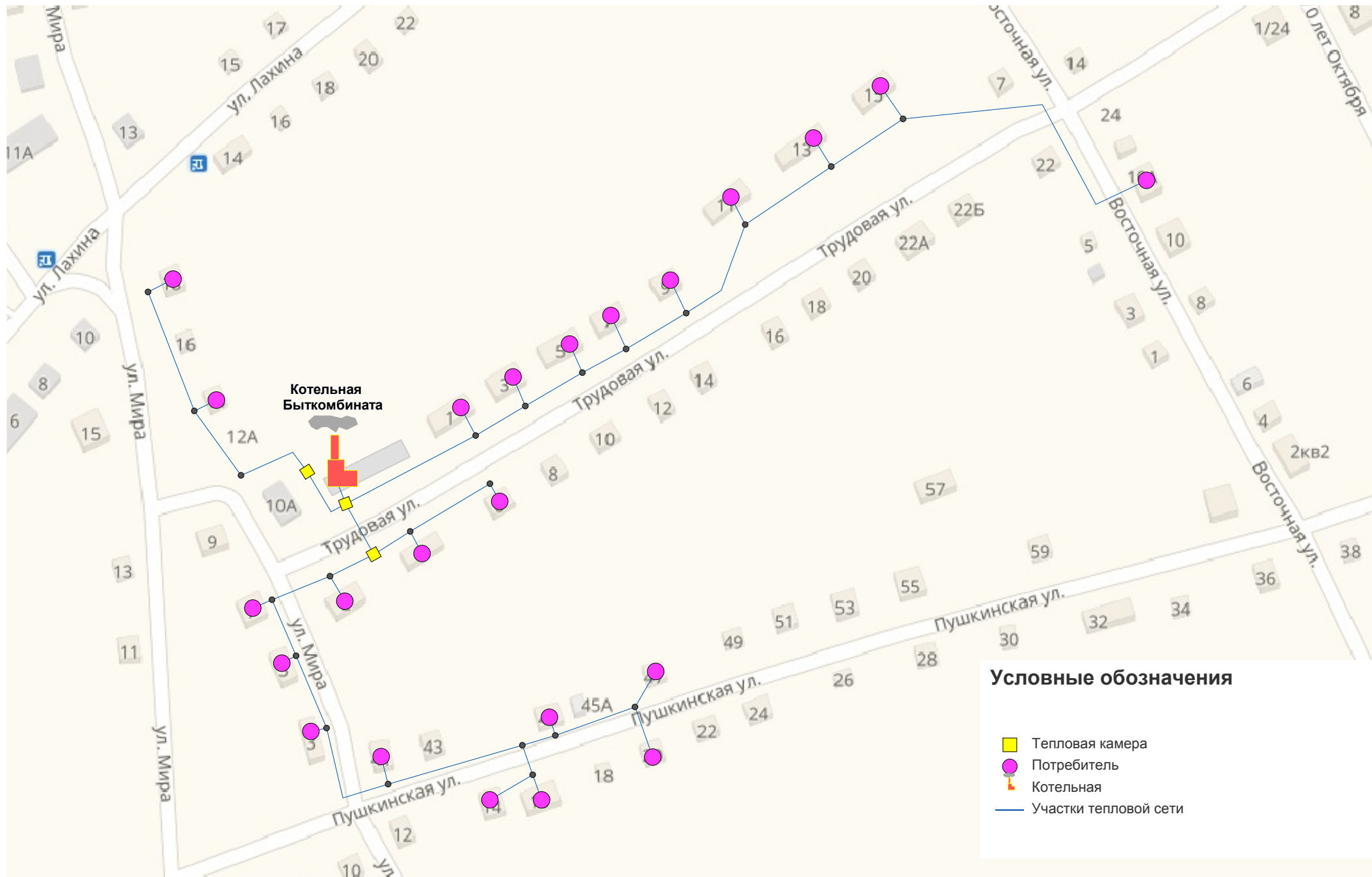
Приложение 5 - Схема тепловой сети котельной "Быткомбинат"
